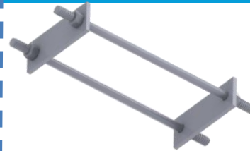
ABRAZADERA EN PLATINAS PARA FIJAR COLUMNA EN CERCHA
